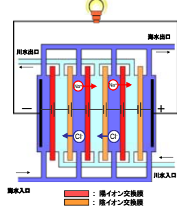
逆電気透析 (RED) の仕組み
