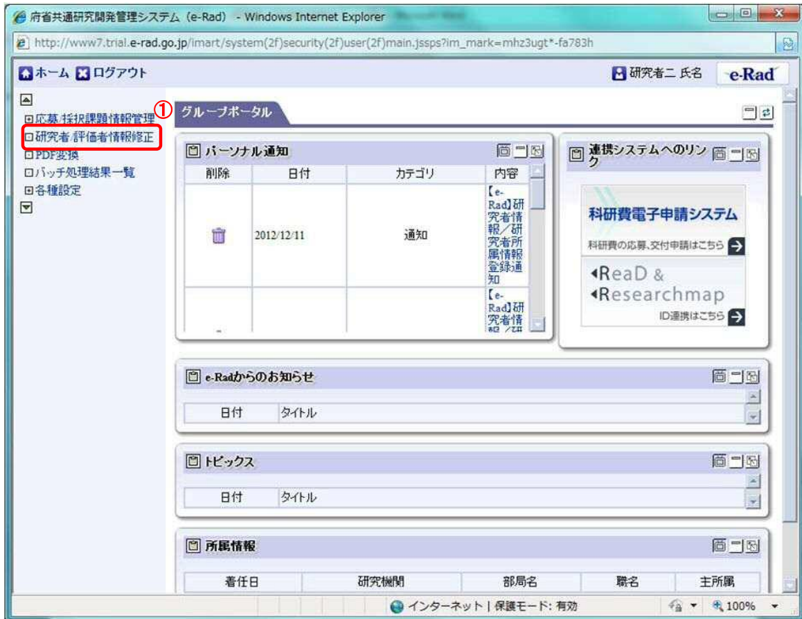
「HOME」画面
